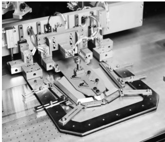
普通换模贴袋机 正常换一套模具安装调试需6-8小时。
