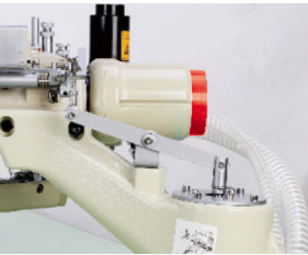
全新设计内置式抬压脚机构 内置式抬压脚，美观静音（可选电动/气动）
