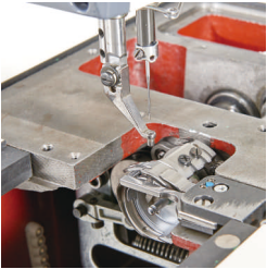
最新剪刀设计 new thread trimmer design
